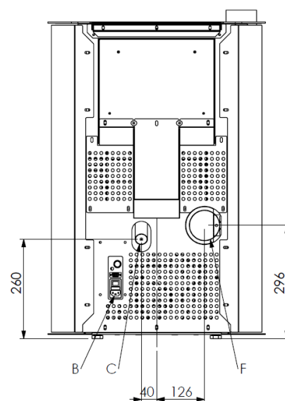
Abmessungen Pelletofen VISION HR
