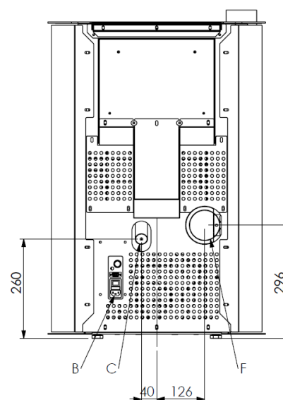
Dimensions du poêle à granulés VISION HR
