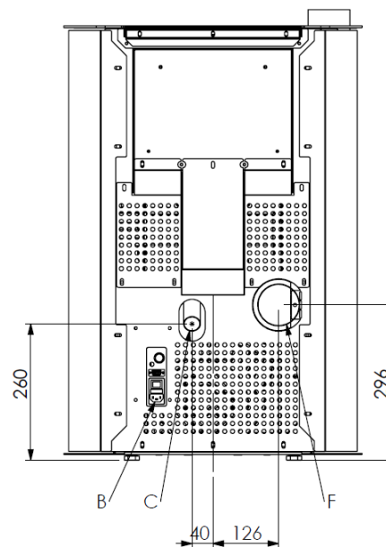
Ingombri stufa pellet VISION HR
