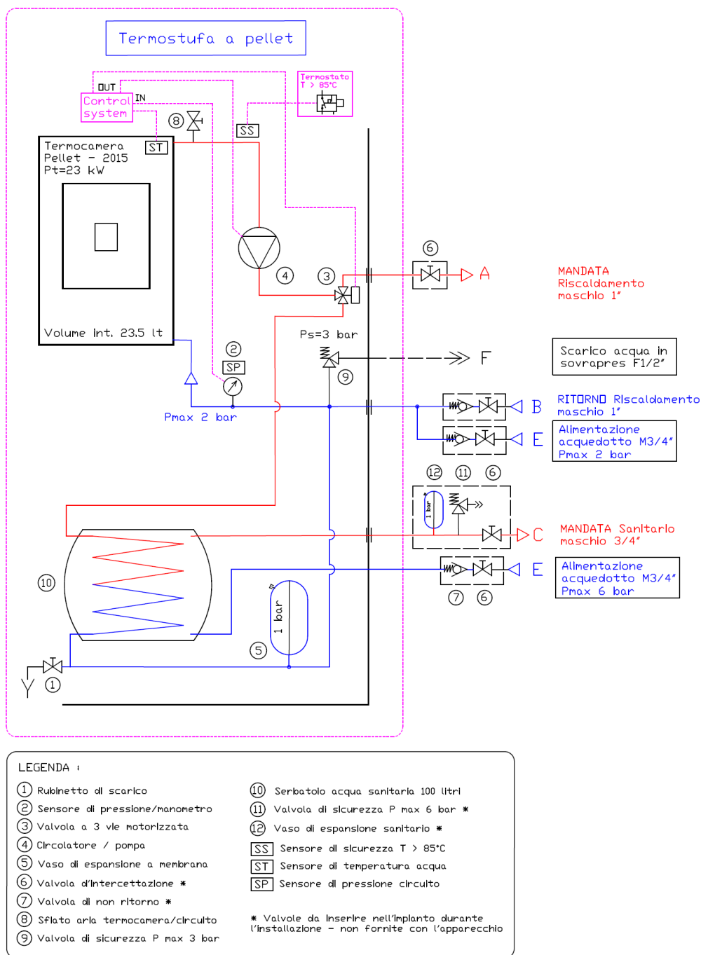
Schema Idraulico Termostufa a pellet 23 kW_04-2015
