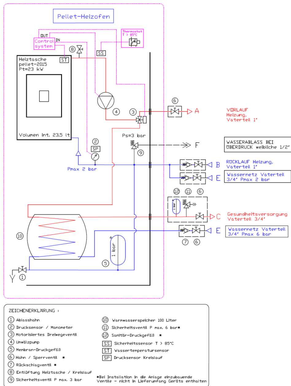
Hydraulischaltplan Pellet-Heizofen 23 kW_04-2015
