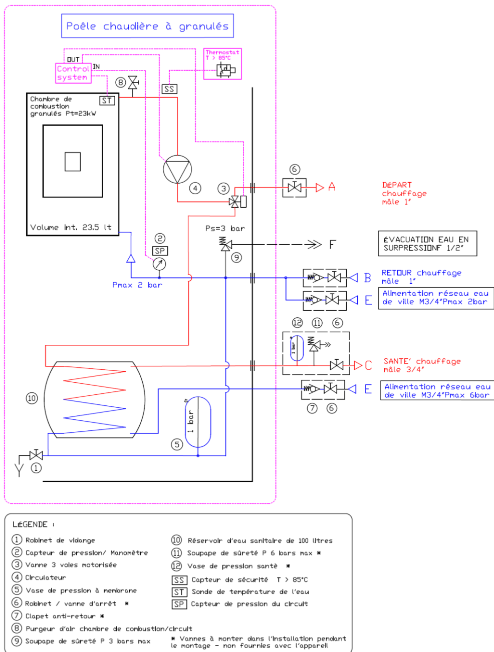
Schéma hydraulique du poêle chaudière à granulés 23 kW_04-2015
