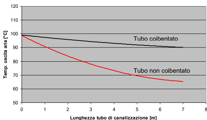
CANALIZZAZIONE ALLA POTENZA NOMINALE ( singola e unica uscita )
