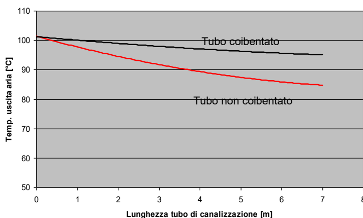
CANALIZZAZIONE ALLA POTENZA NOMINALE ( singola e unica uscita )
